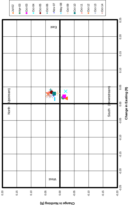
Monitoring Point SM151 (subset)
