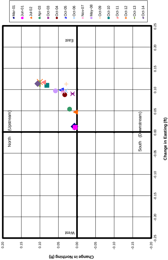
Monitoring Point SM127 (subset)
