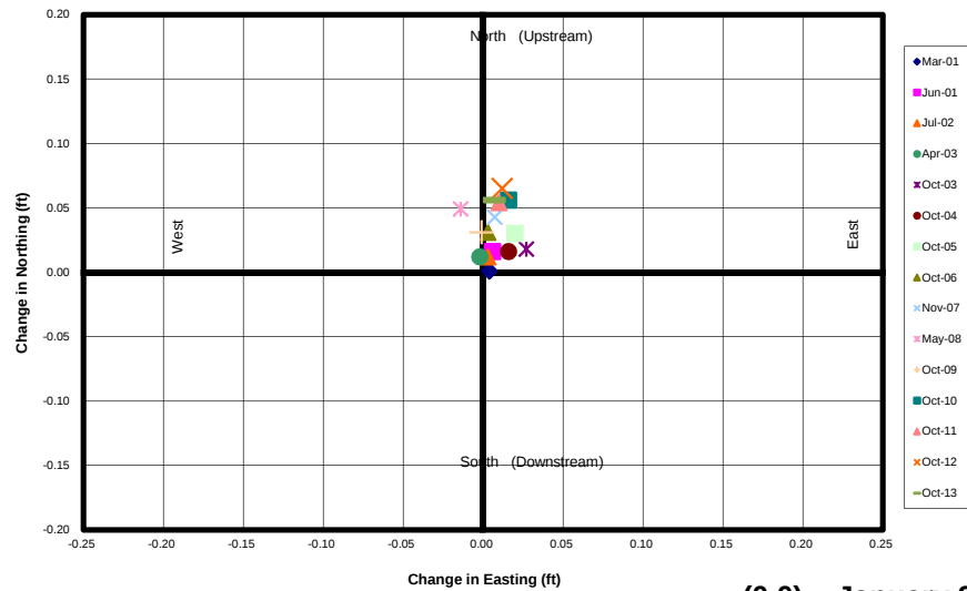
Monitoring Point SM177 (subset)
