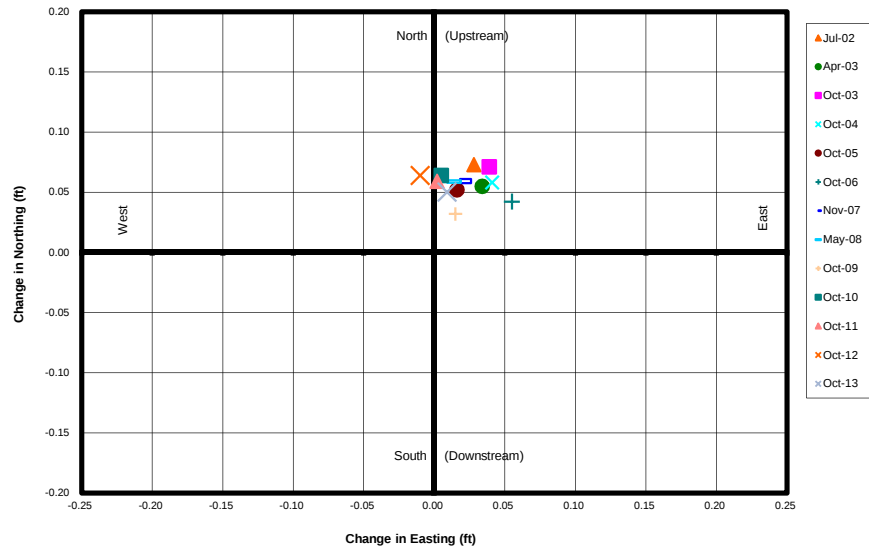
Monitoring Point SM104 (subset)
