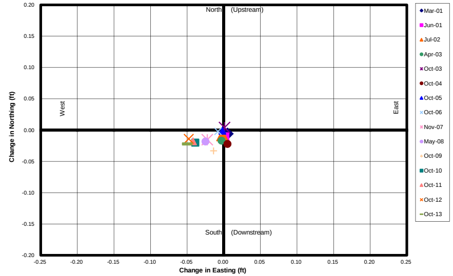
Monitoring Point SM105 (subset)
