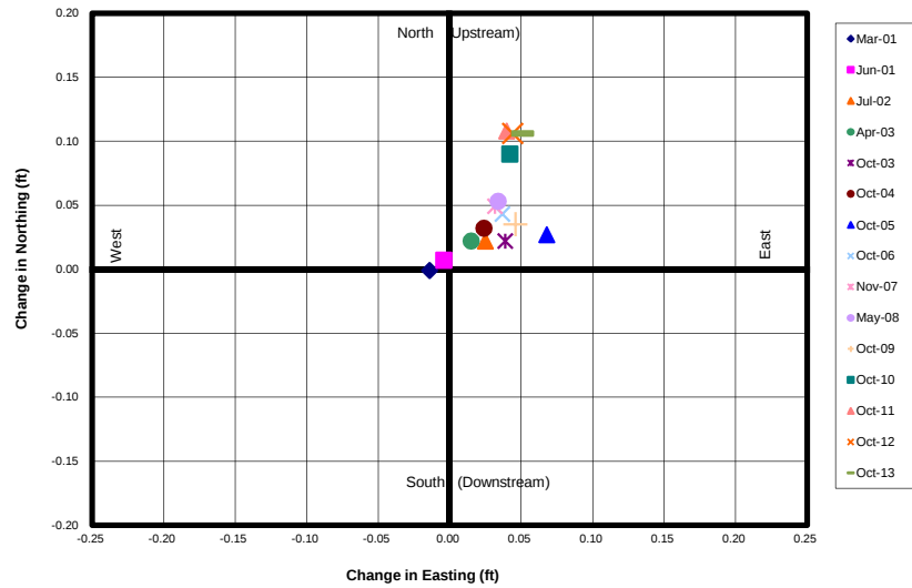
Monitoring Point SM161 (subset)
