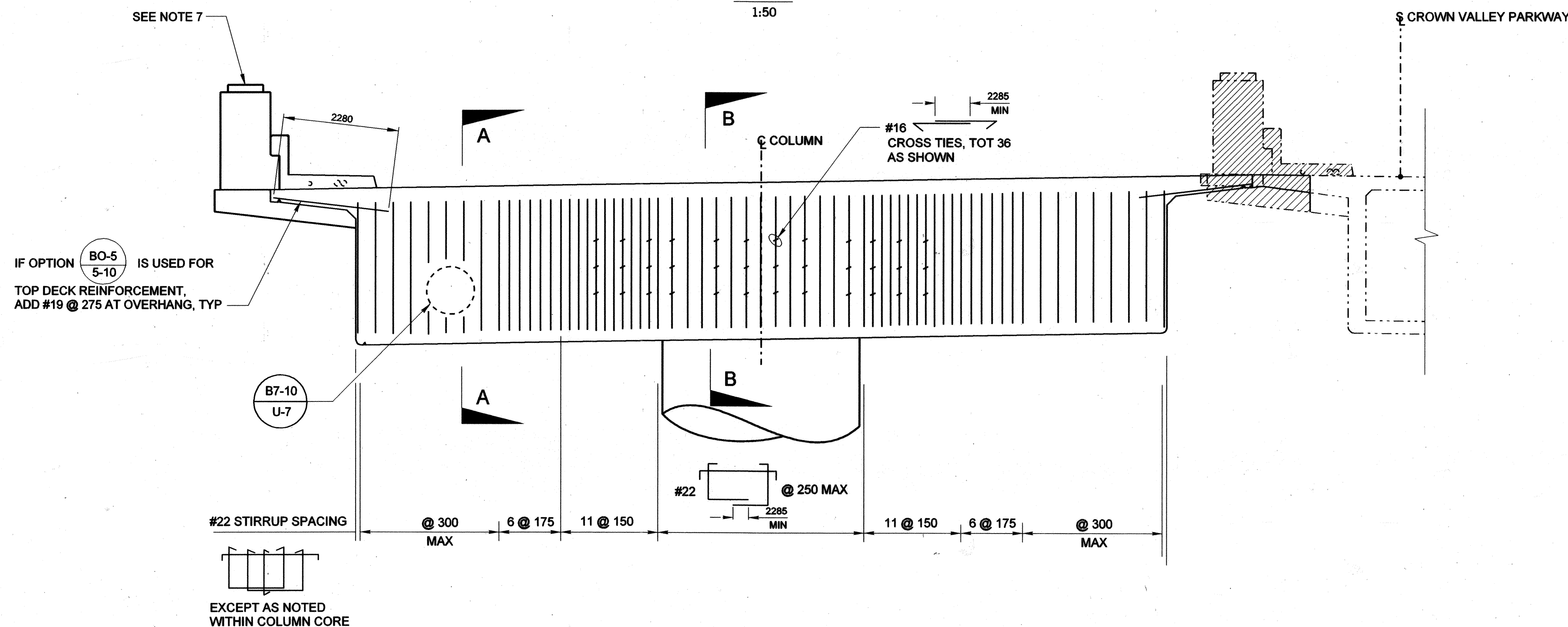
ELEVATION 1:50
