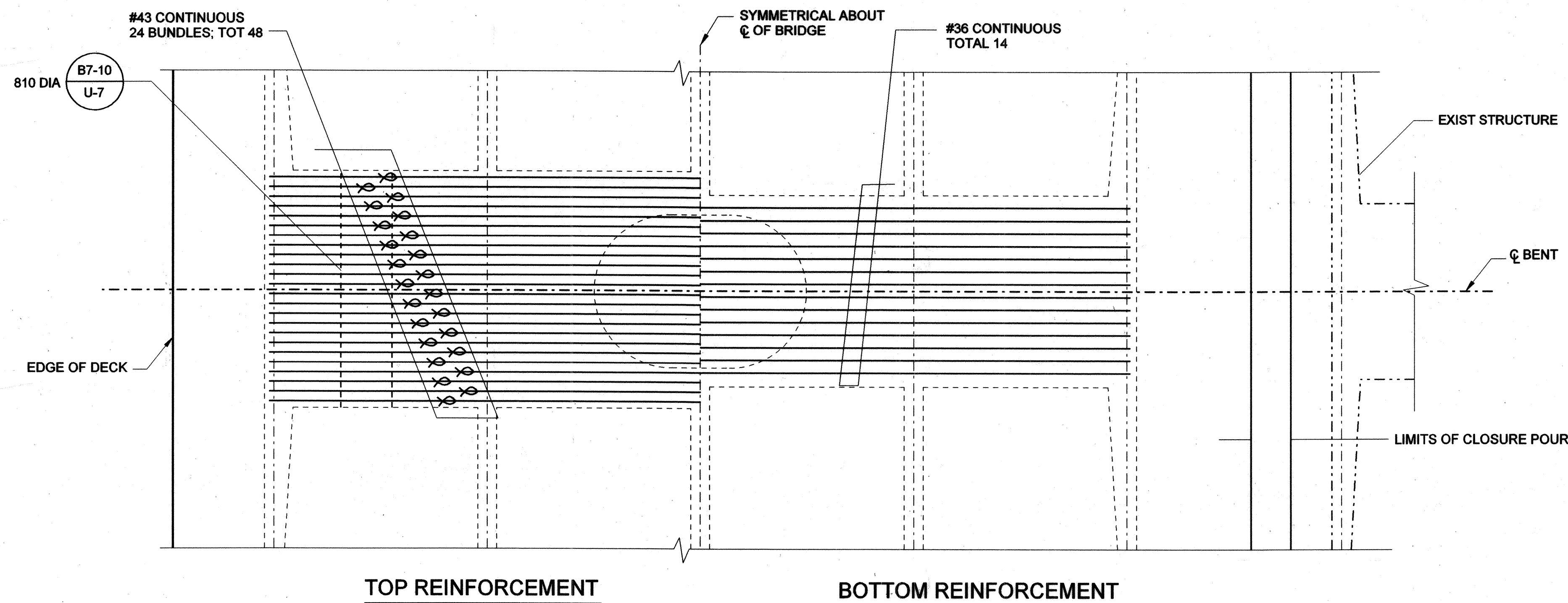
PLAN 1:50
